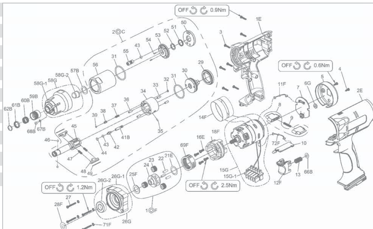
Despiece de la pistola SPPW-15
