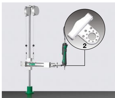
Braccio Cartesiano BCA
